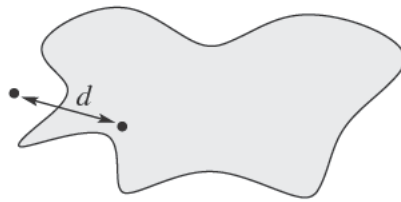
Fig. 23.11. Gaussian sampling
