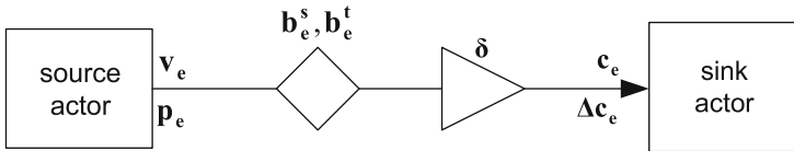
Fig. 5.7 Single WDF edge
