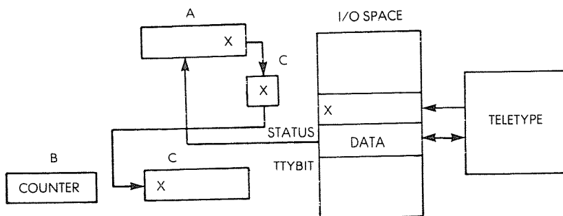
Fig. 6.15: Teletype Input
