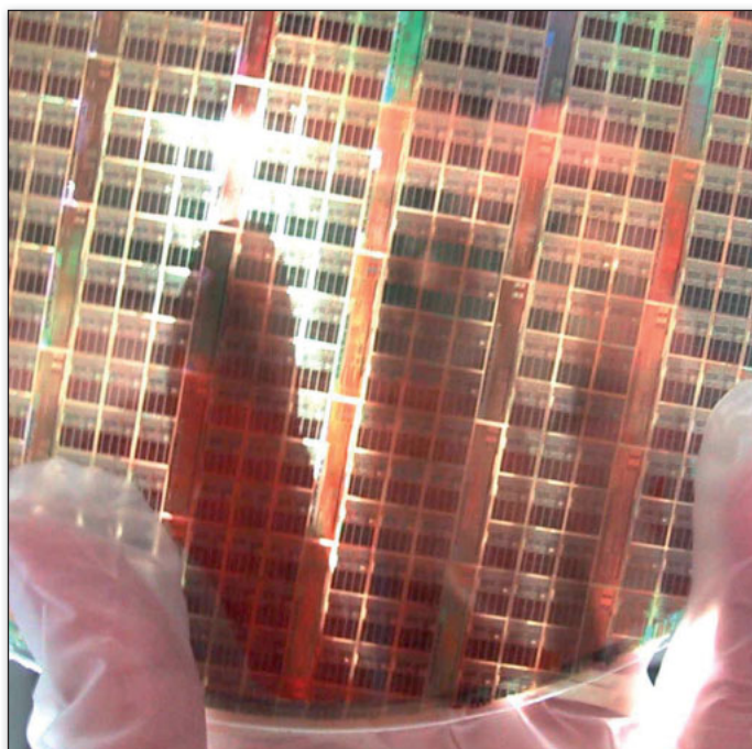
Chipskex. Så här ser det ut i IBM:s labb, när chipset sätts ihop till en "wafer".
